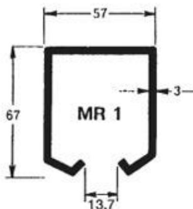
Tipo per carrelli grandi peso al m kg 5,000
