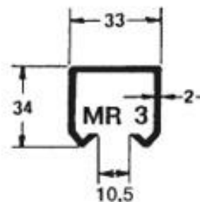
Tipo per carrelli mignon peso al m kg 1,774
