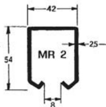
Tipo per carrelli piccoli peso al m kg 3,180
